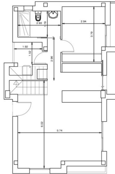
PLANTA BAJA
