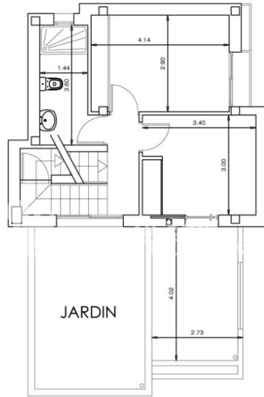
PLANTA 1ª
