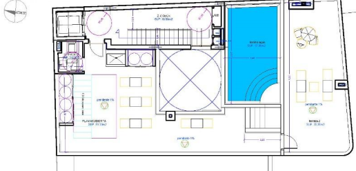
ESQUEMA DISTRIBUCIÓN
