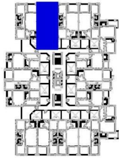
PLANTA SEGUNDA
