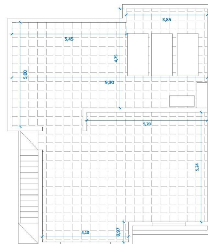
SOLARIUM MODELO A
