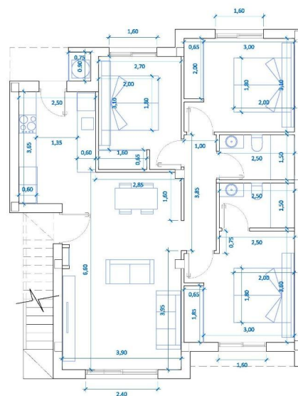
PLANTA MODELO A
