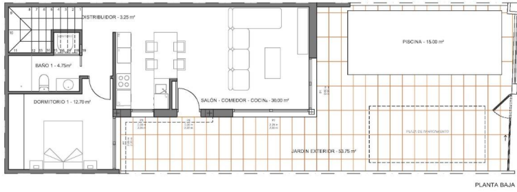
PLANTA BAJA
