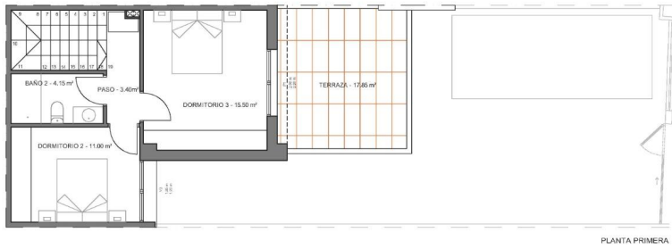
PLANTA PRIMERA
