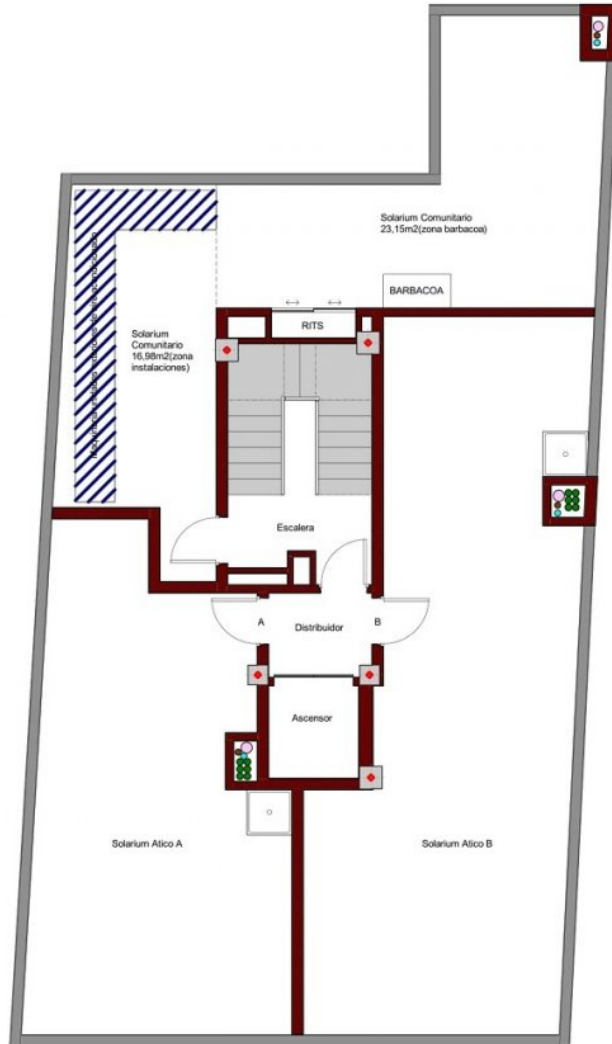
PLANTA CUBERTA
