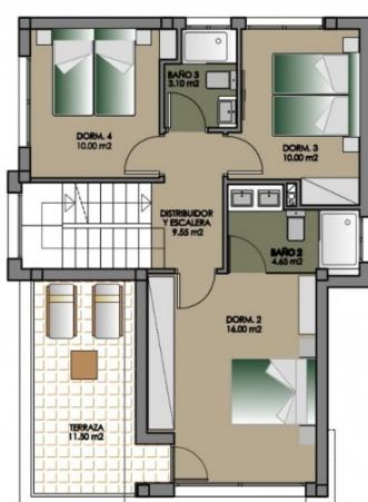
PLANTA PISO
