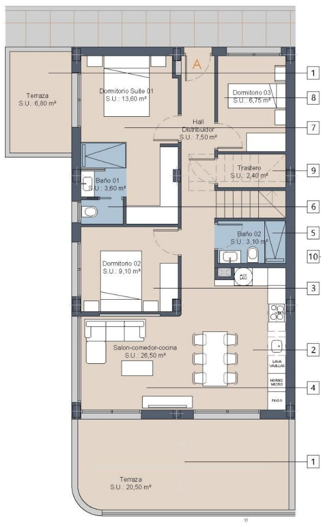
0 0,5 1 2 3 4 5 PLANTA PRIMERA
