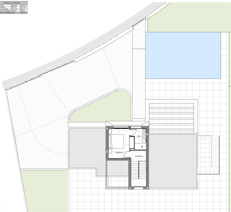
PLANTA PRIMERA
