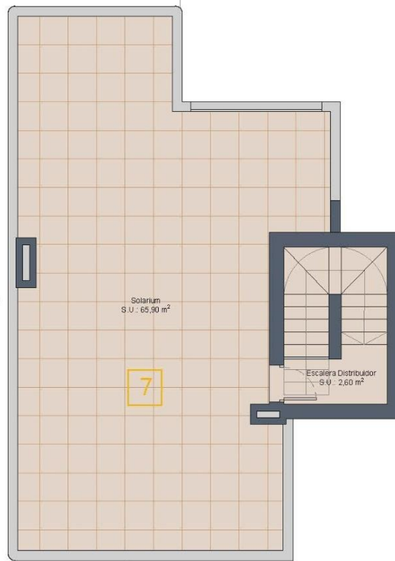
PLANTA SOLARIUM
