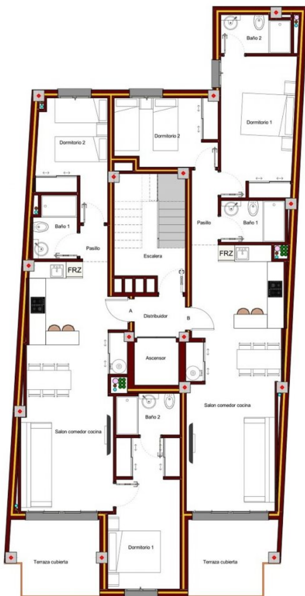
PLANTA TIPO
