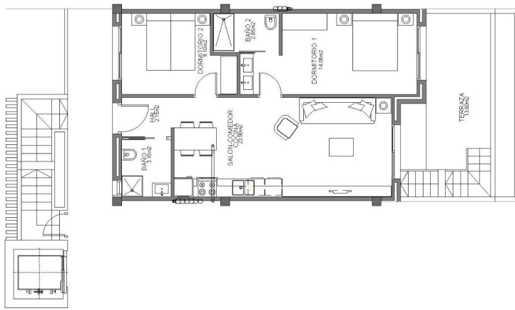
Planta Segunda
