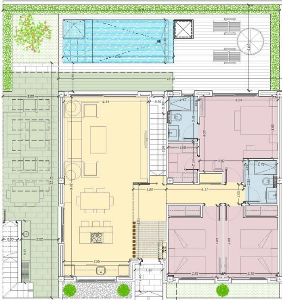
PLANTA BAJA
