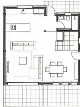
PLANTA BAJA
