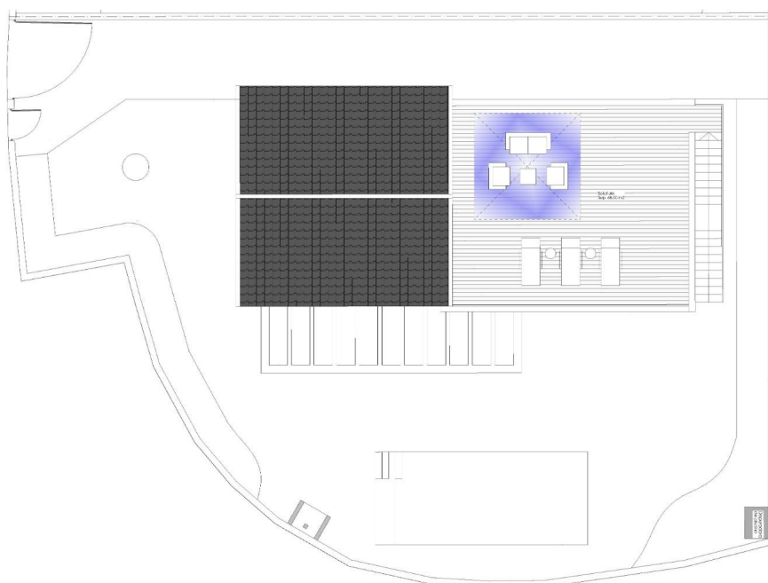
PLANTA SOLARIUM
