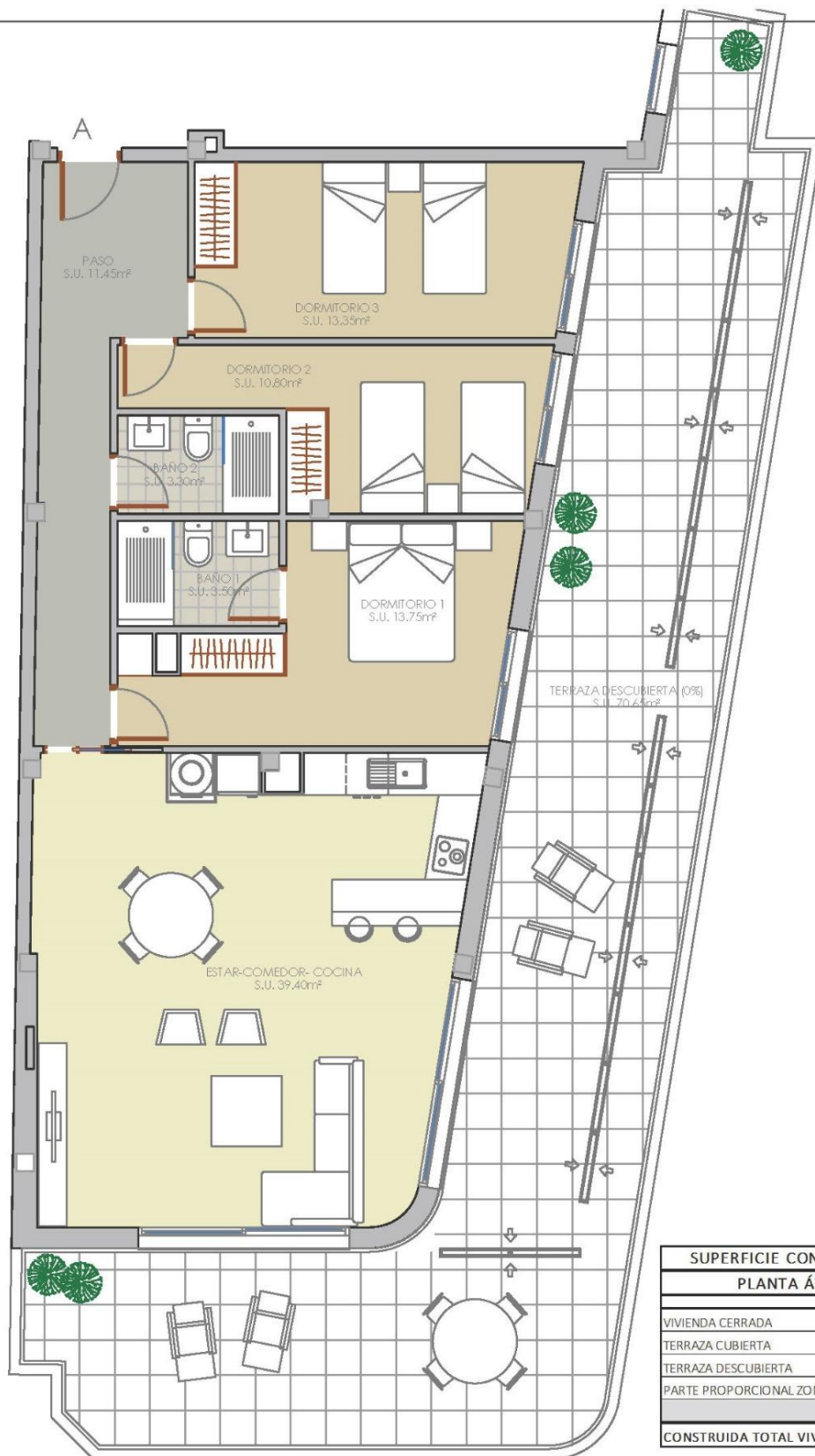
PLANTA ÁTICO
