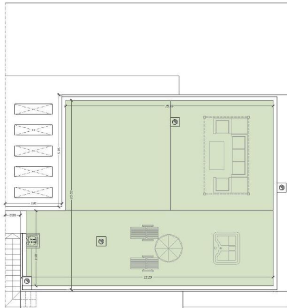
PLANTA CUBIERTA-SOLARIUM
