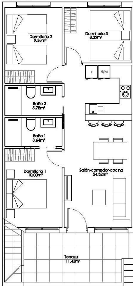
Planta Vivienda
